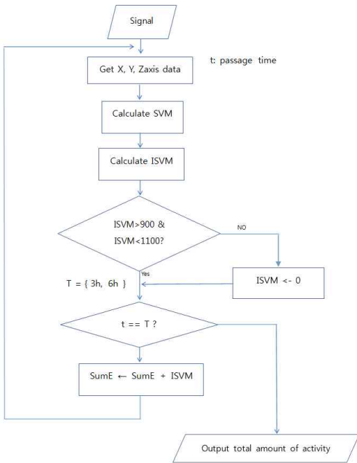
그림 4. 알고리즘 흐름도 Figure 4. Flow chart of algorithm
