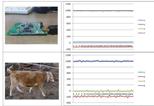
그림 5. 장소별 3축 가속도 센서 그래프 Figure 5. The graph of Measured data with 3-Axis sensor in different place
