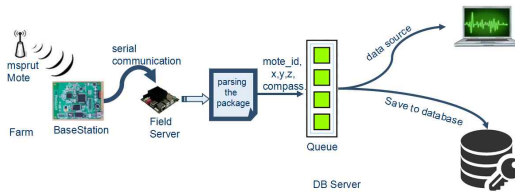
그림 2. 시스템 구성도
