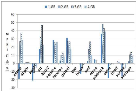
그림4. 분할 그룹 수에 대해 LRU보다 제안 방법의 MPKI 감소율 Figure 4. MPKI reduction rate over LRU of proposed scheme for the number of divided groups
